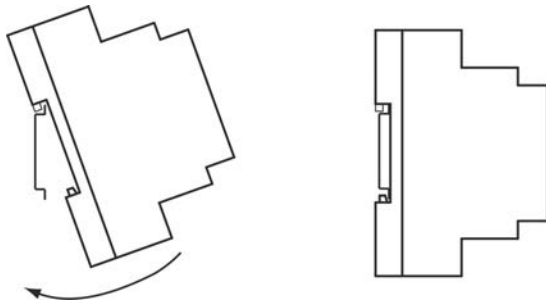
Figur 6. Installation af idOil-kontrolenheden
