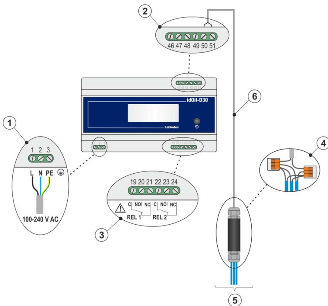
Figur 14. Tilslutning med en tre-sensorkabelkonnektor
