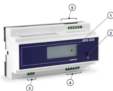
Figur 27. idOil-kontrolenhedens funktioner
