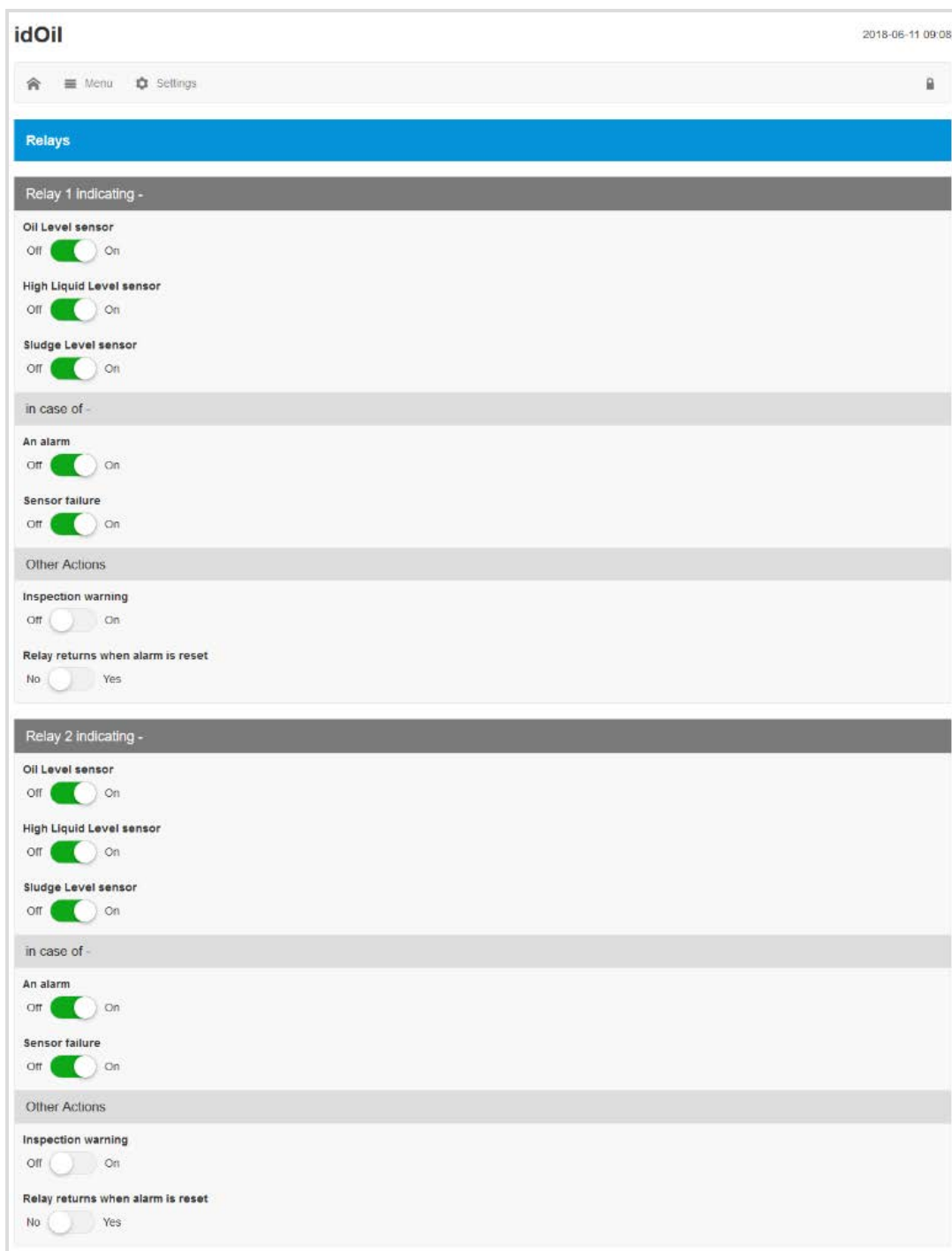
Figur 40. Relæindstillinger
