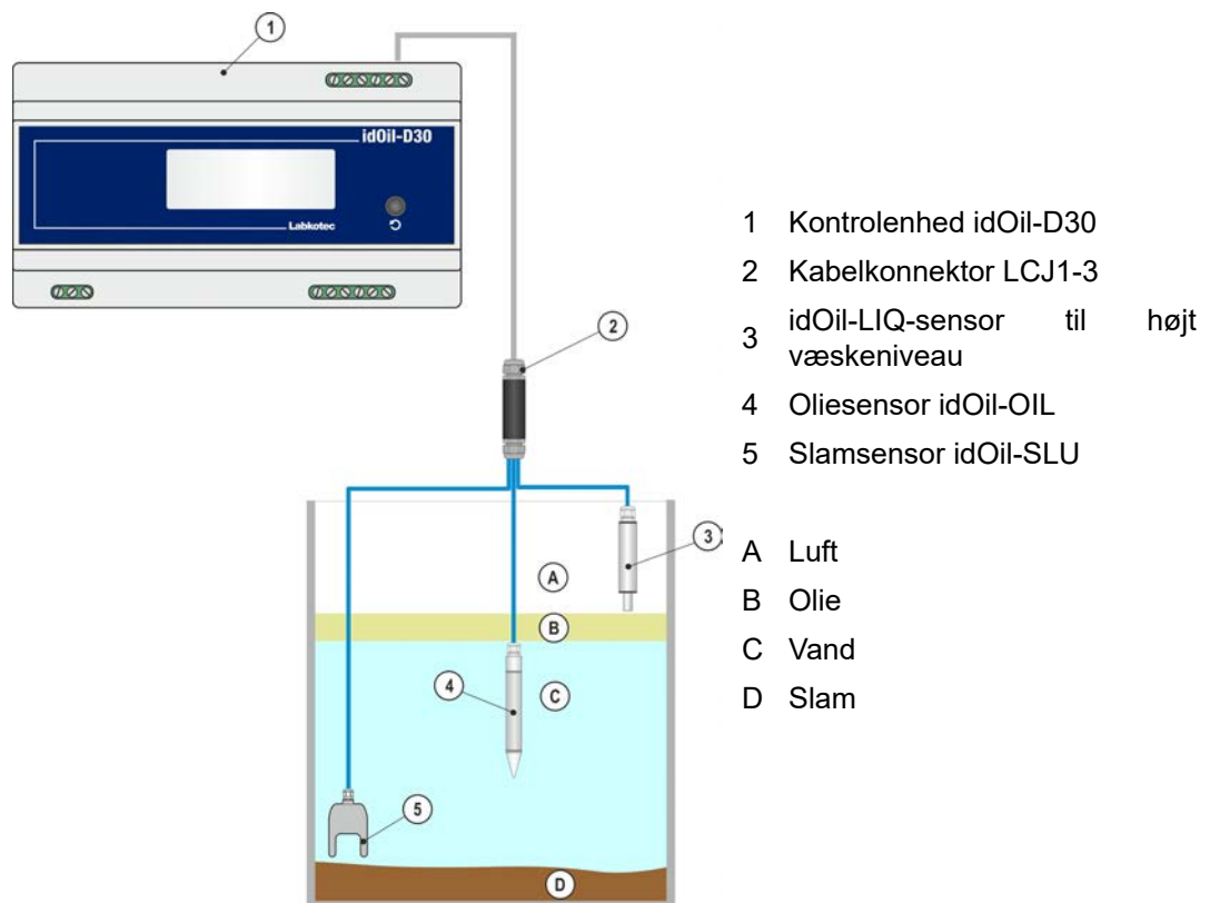
Figur 1. Systembeskrivelse; idOil-kontrolenhed, sensorer og kabelforlængelse
