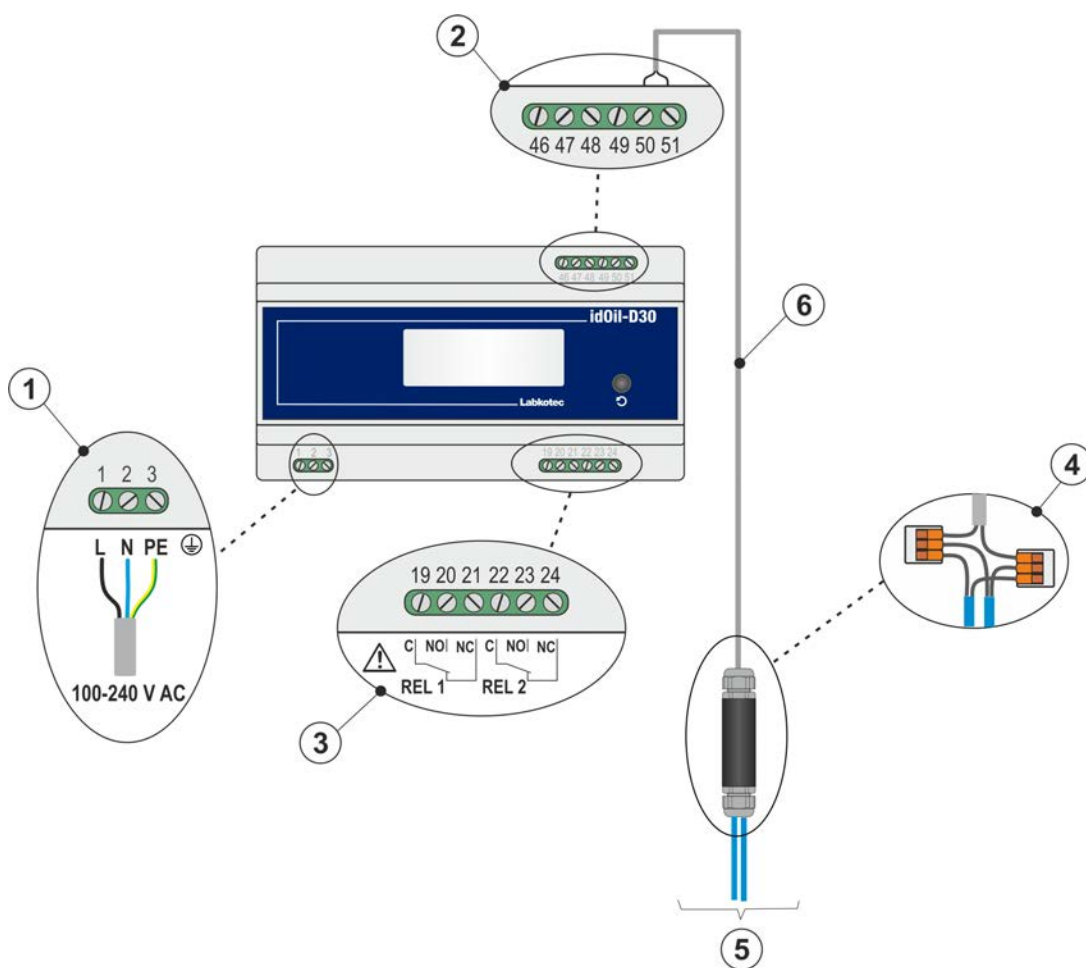
Figur 13. Tilslutning med en to-sensorkabelkonnekter
