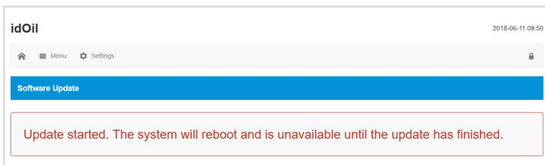
Figur 44. Softwareopdatering startet
