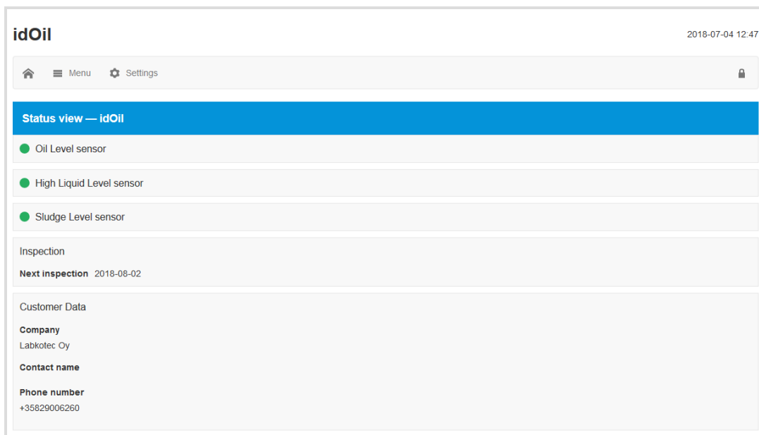
Figur 28. Hjemmeskærm
