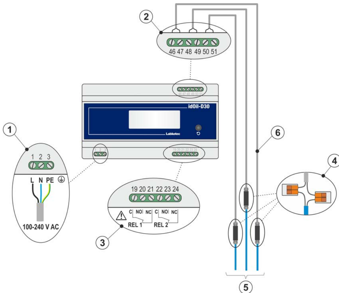
Figur 12. Tilslutning med en enkeltsensorkabelkonnekter
